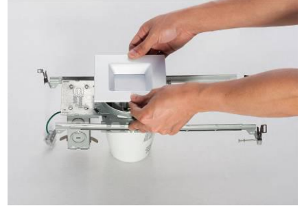
Step3: Insert LED trim.
