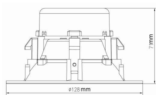
Size : \Phi 128 \times 71 \text{mm} (5.04 x 2.8")
